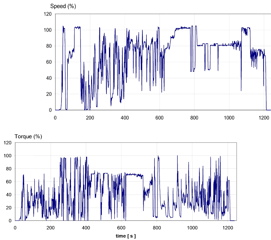
그림 3. NRTC 싸이클
